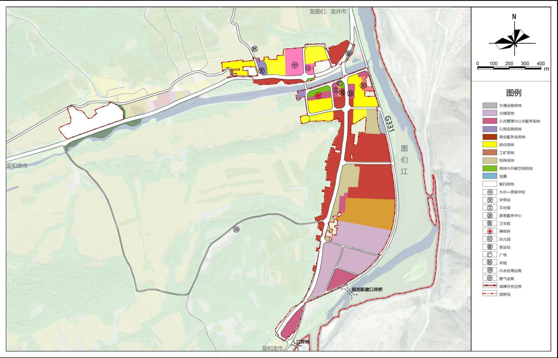
镇区-用地布局规划图
